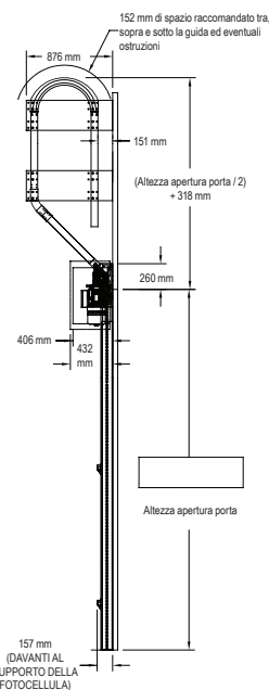
ALZATA AVVOLGIMENTO POSTERIORE
