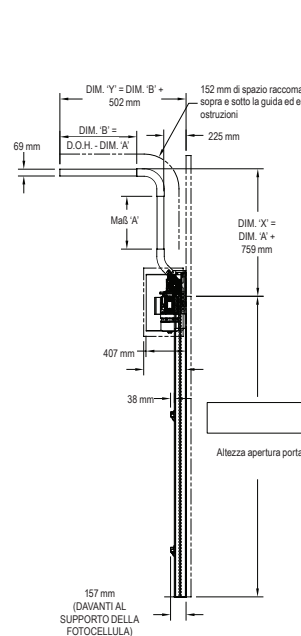
ALZATA VERTICALE ALTA
